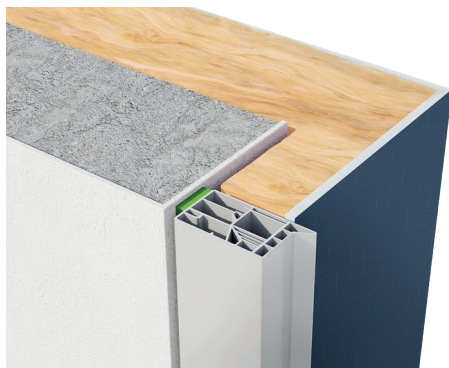
Figure 3 : Tunnel au nu intérieur - ITE avec retour
