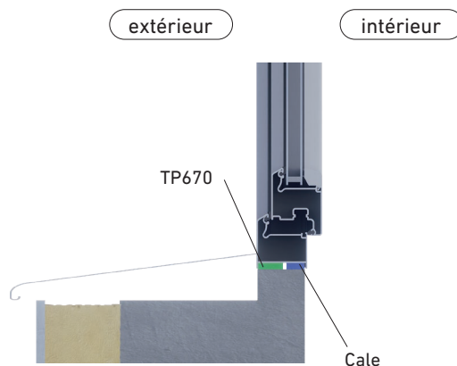
Figure 7 : Pose en partie basse avec rejingot
